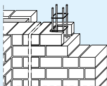
Aussteifungsstütze mit KS-U-Schalen
