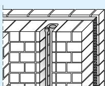
Lotrechter Schlitz mit KS-U-Schalen
