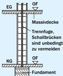
Schnitt
