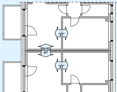
Doppel- und Reihenhäuser mit zweischaligen Haustrennwänden
