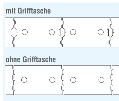
KS-Mauerwerk ohne Stoßfugenvermörtelung (Draufsicht)
