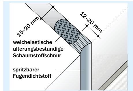
Bild 48 Dehnungsfuge mit spritzbarem Fugendichtstoff
