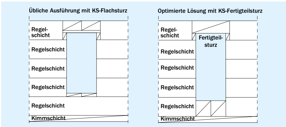
Bild 9 Bei der Festlegung der Kimmerschichthöhen sollten Brüstungshöhe und Sturzaufleger berücksichtigt werden.
