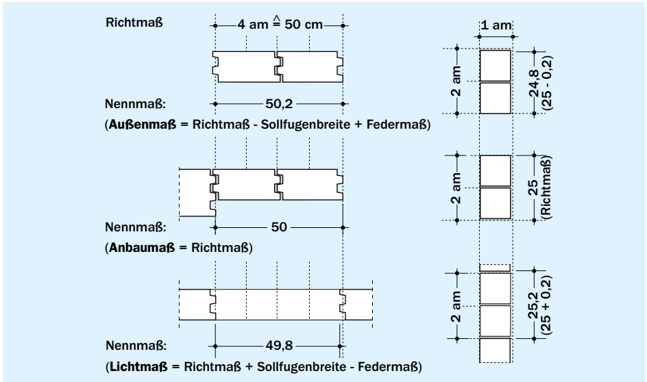
Bild 5 Richtmaße und Nennmaße für Bauweise ohne Fuge (Mauerwerk aus Steinen mit Nut-Feder-System)
