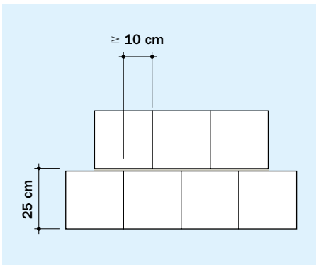
Bild 7 Mindestüberbindemaß l_{ol} für KS-Plansteine
