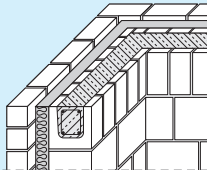
Ringbalken mit KS-U-Schalen
