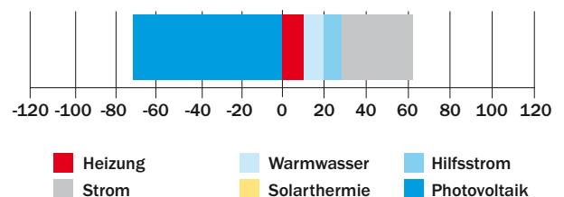
Primärenergiebilanz (Bereiche Heizung, Warmwasser und Hilfsstrom weisen eine Plusenergiebilanz auf)
