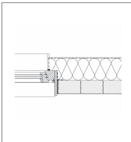
Fenster - Leibung
