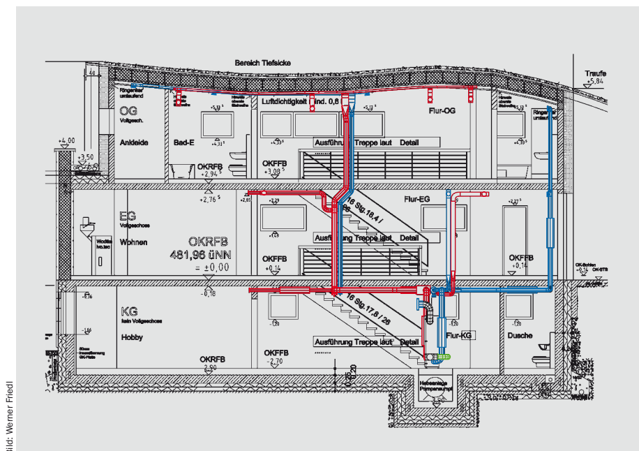
Schnitt mit eingezeichneter Lüftungsplanung
