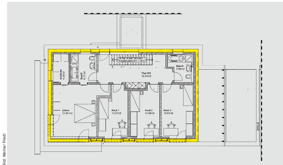
Grundriss OG
