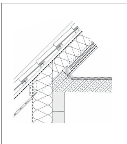
Traufe – Außenwand
