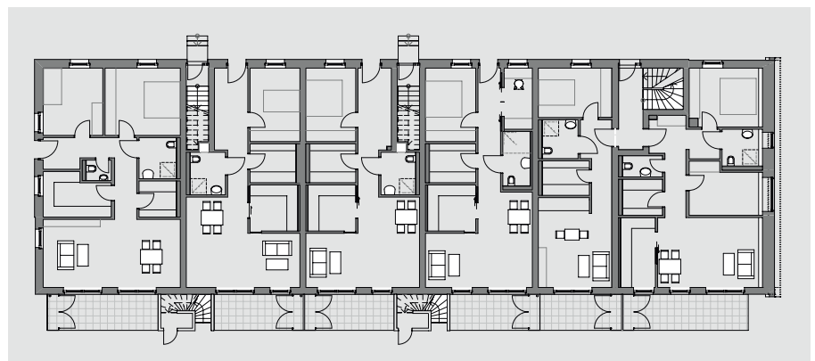
Regelgrundriss
