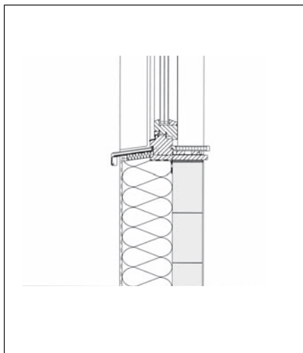
Fenster - Brüstung
