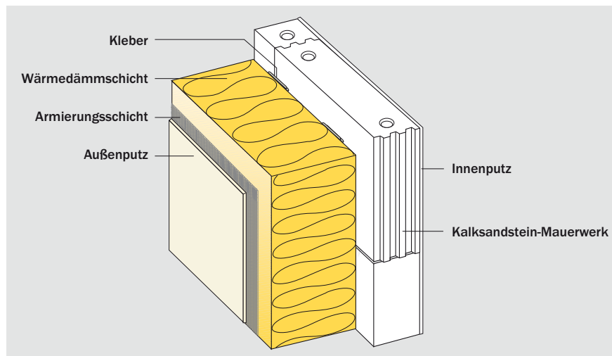
Wärmedämmverbundsystem (WDVS) auf Kalksandstein-Mauerwerk
