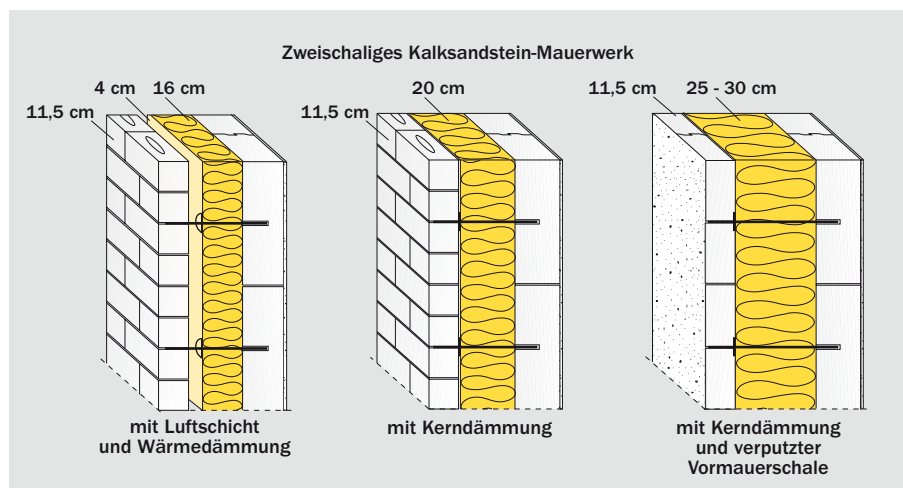
Konstruktionsmöglichkeiten für zweischaliges Mauerwerk
