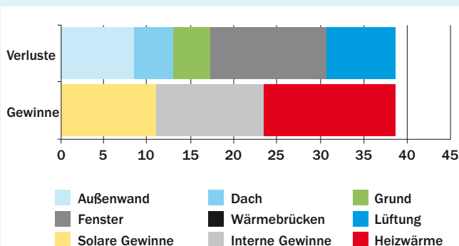
Energetische Bilanzierung des Heizwärmebedarfs: Gewinne und Verluste [kWh/(m 2 a)]
