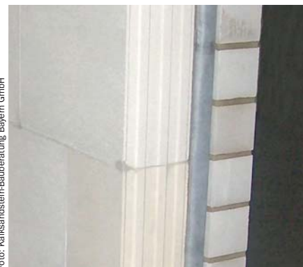
Anschluss Verblendmauerwerk
