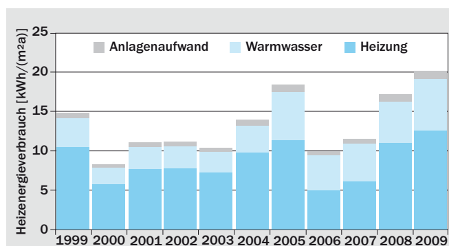
Heizenergieverbrauch Einfamilien-Passivhaus Erlangen, Dorfmeisterweg
