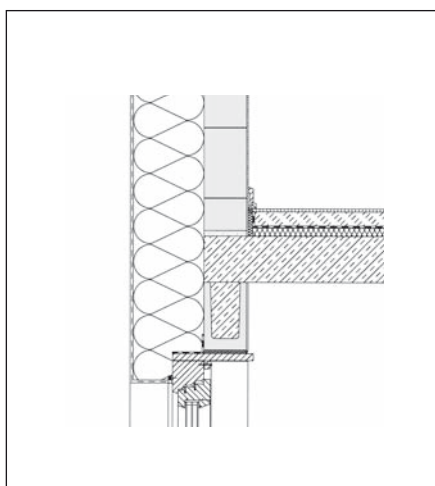
Fenster - Sturz
