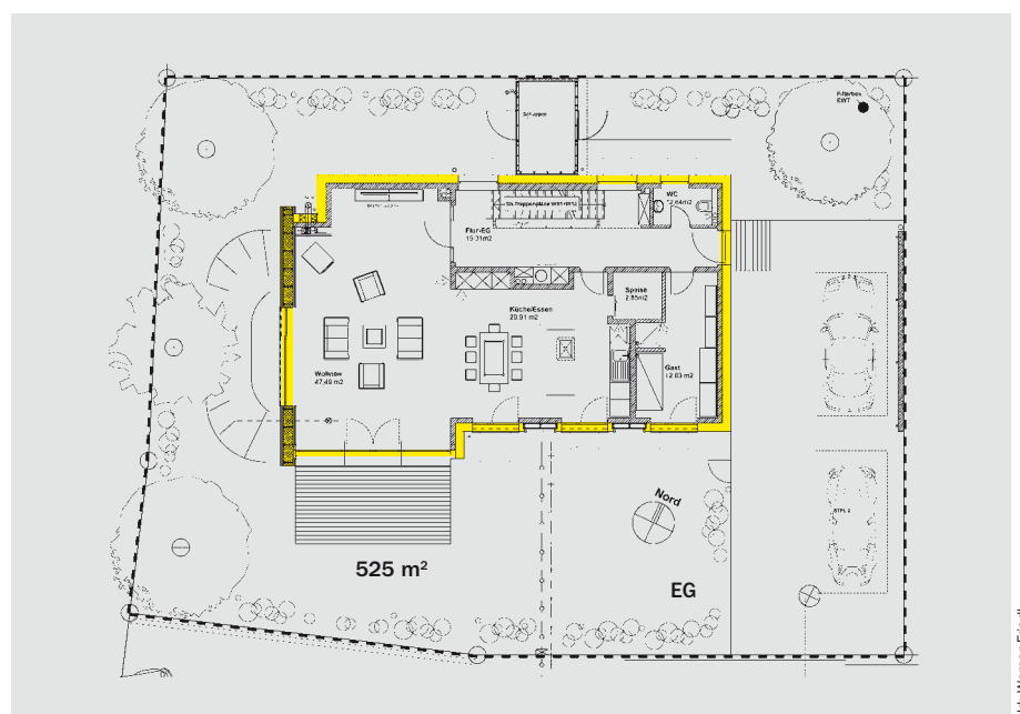
Grundriss EG
